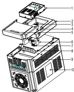
2-3. ábra Termék struktúradiagram
