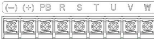
3-7 ábra főáramkör kivezetései – 3 fázis – 30-37kW-ig
