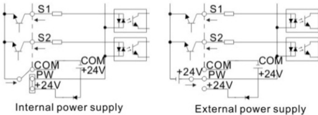
3-13. ábra NPN módok
